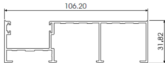
TRIPLE REVERSIBLE FRAME JAMB AL628
