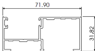
REVERSIBLE FRAME JAMB AL615
