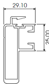
H/DUTY INTERLOCK AL620
