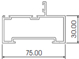
VISTAFOLD JAMB AL563
