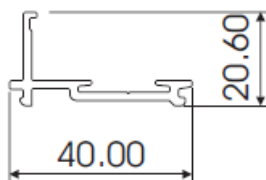
R4 FILLER AL016
