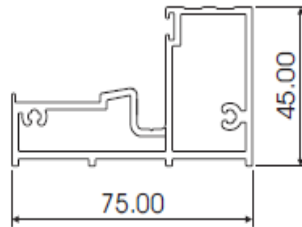
VISTAFOLD SILL AL562
