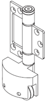
BOTTOM ROLLER
