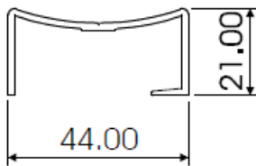
PIVOT DOOR END STYLE AL451
