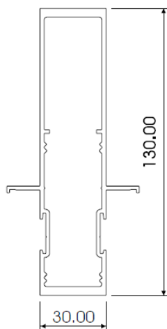
K130 2 LIP AL857
