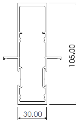
K105 2 LIP AL380
