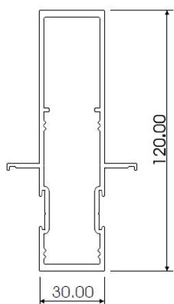
K120 2 LIP AL345
