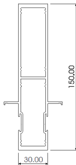
K150 2 LIP AL023
