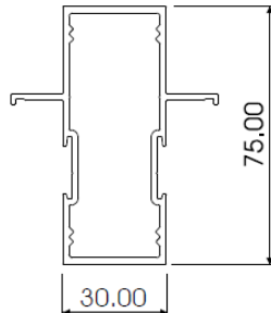
K26 2 LIP AL002
