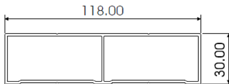
DOUBLE BOX JAMB AL362
