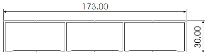
TRIPLE BOX JAMB AL634
