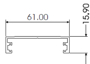
JAMB ADAPTOR AL369
